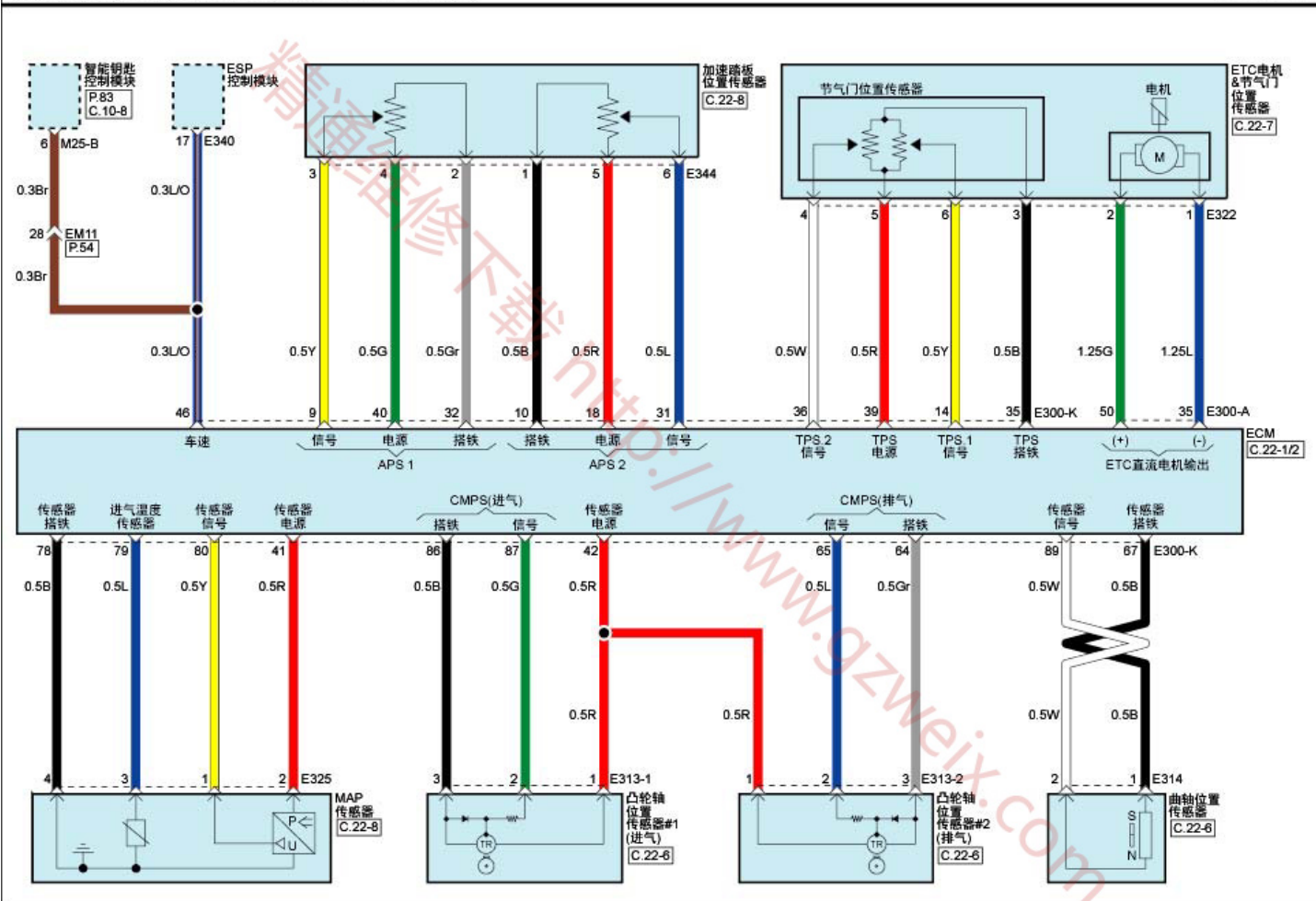
发动机控制系统(G4FJ : GAMMA 1.6L T-GDI)(6)
